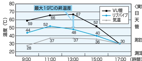
参考：リブパイプ屋外曝露による昇温実験結果
